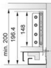
Montaje Mínimo
