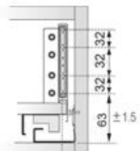
Montaje frontal
