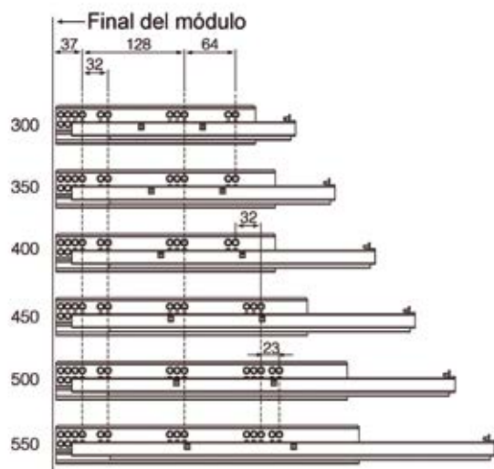
Montaje Mínimo
