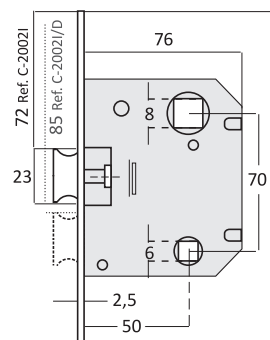
Picaporte 70 mm descentrado. / Off center (70 mm)
