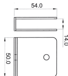
K17U SS 304 Pinza de sujeción lateral para panel, en U. Acero inoxidable. Clamp side union. Stainless steel. Union côté pince. Acier inoxydable.
