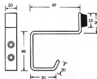
K17U SS 304 Pinza de sujeción lateral para panel, en U. Acero inoxidable. Clamp side union. Stainless steel. Union côté pince. Acier inoxydable.
