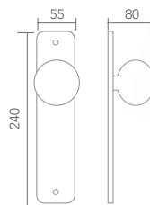
ATI-138 Placa pomo fijo Inoxidable
