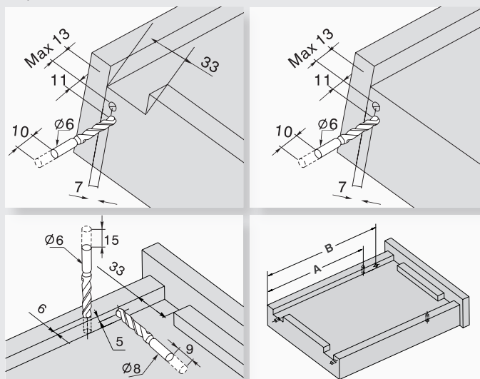
Preparación del cajón (mm)
