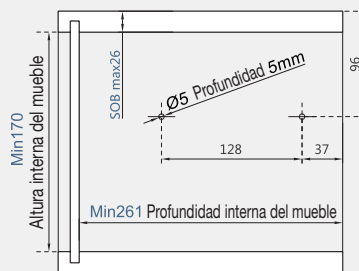
Cotas de los posicionadores y espacio requerido
