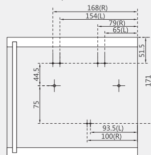
Cotas de los tornillos de 4 x 38 mm. para fijar el elevador.
