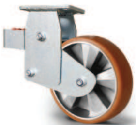
placa fija con amortiguador
